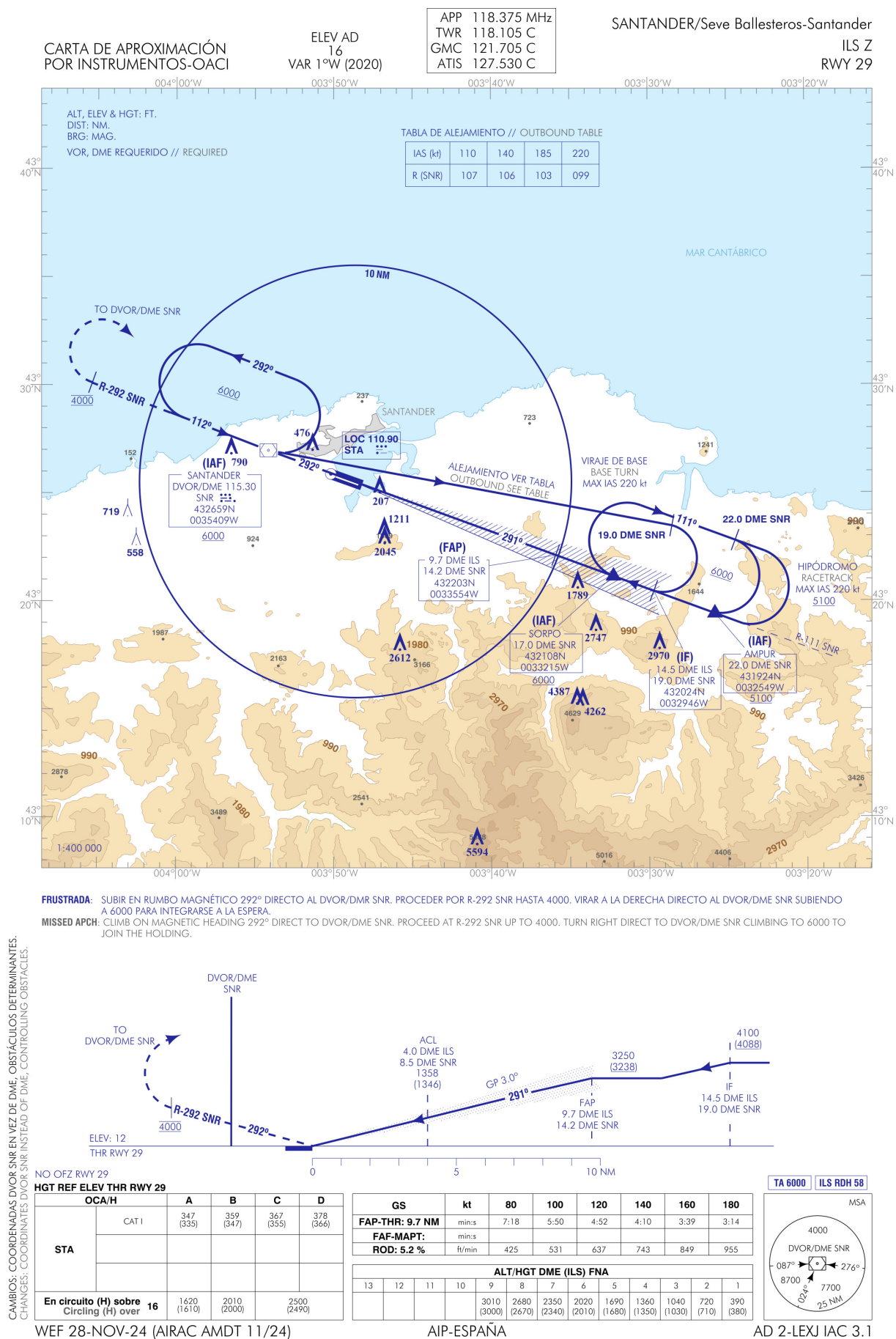
Figura 3.23: Aproximación por instrumentos a LEXJ RWY 29 procedimiento ILS [Fig28].
